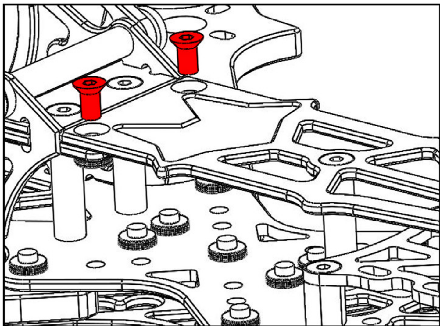
M3x6mm tête fraisée X2
