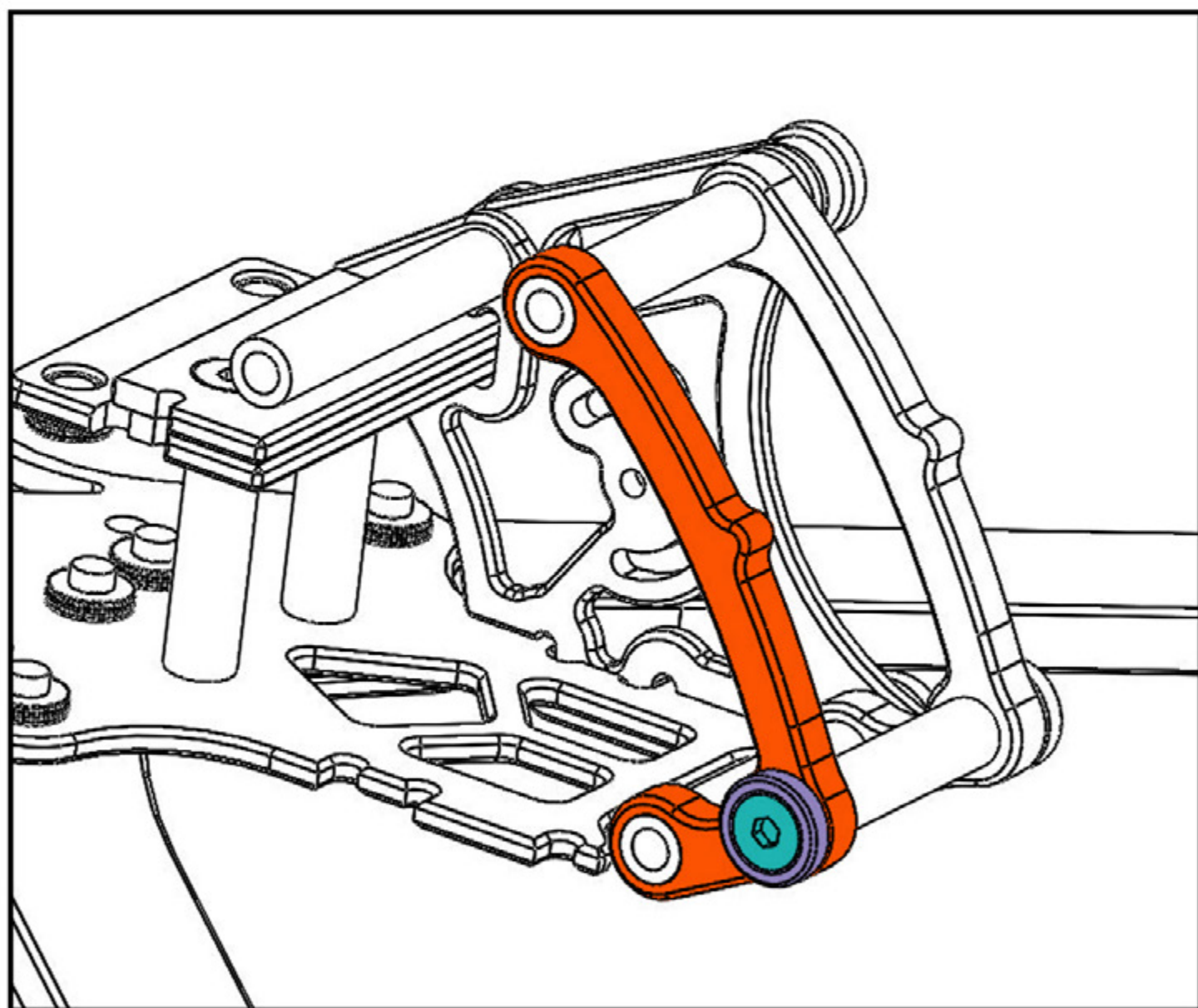
M3x10mm tête fraisée X1
