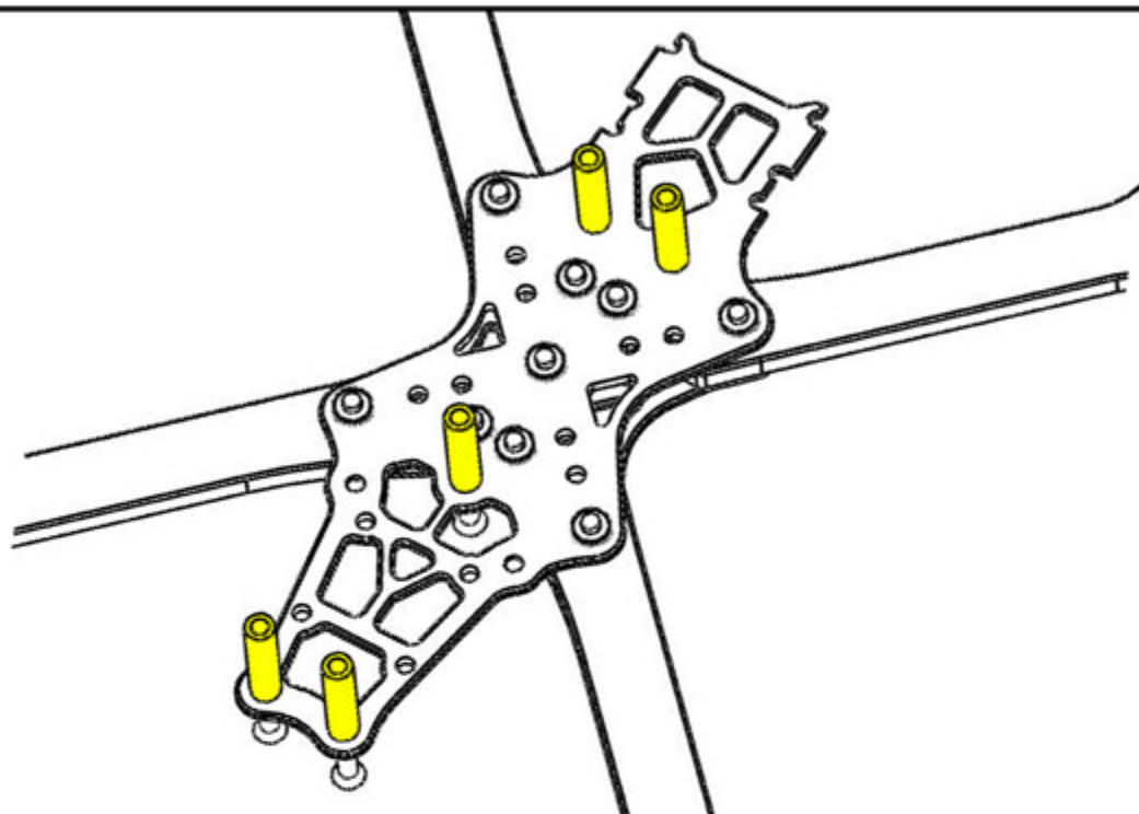
vis M3x8mm tête fraisée X5
